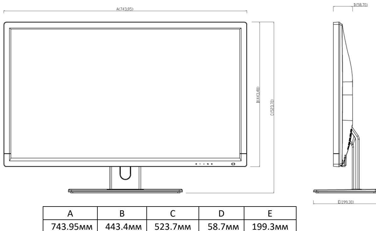
Рисунок 4-1 Размеры устройства
