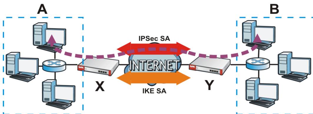
Figure 375 VPN: IKE SA and IPSec SA
